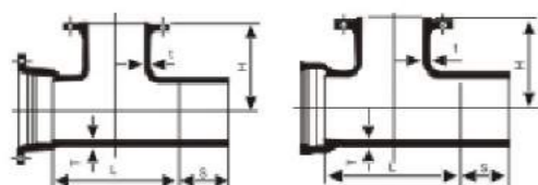
规格DIMENSIONS(PN16)
